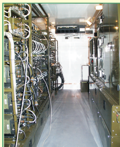
Widok AWRS od wewnątrz
